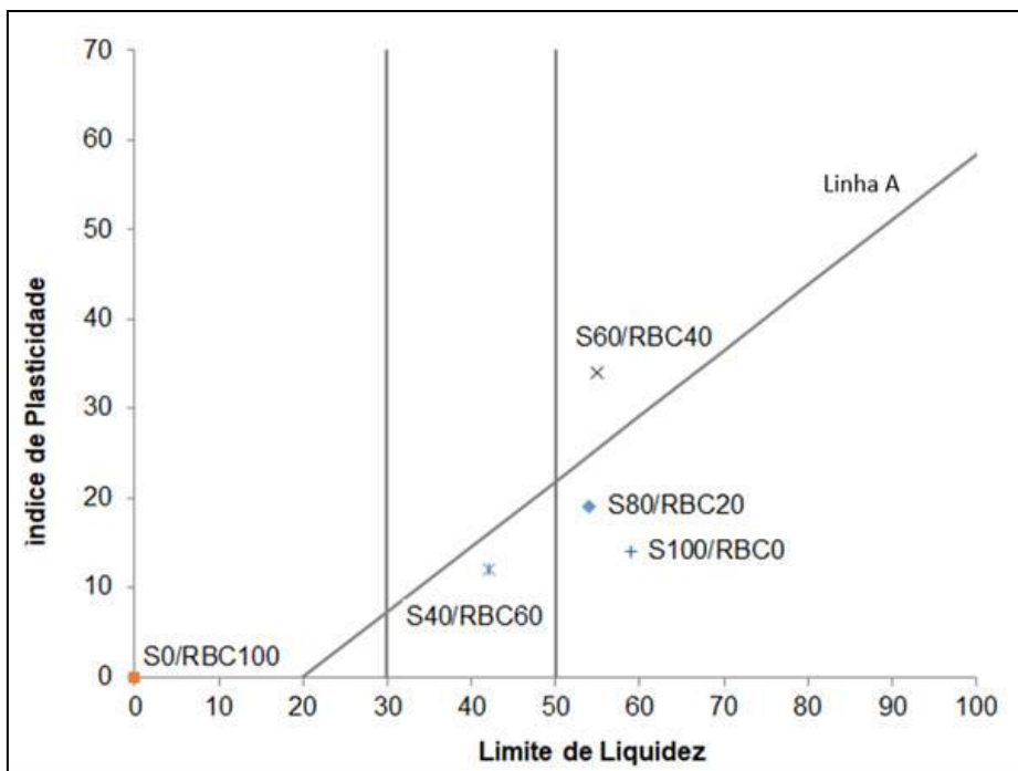
Figura 5 - Localização das misturas de solo e RBC no gráfico de plasticidade de Casagrande
