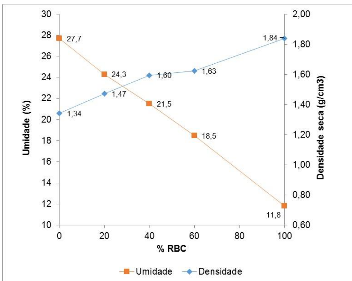
Figura 8 - Umidade ótima e densidade máxima seca para misturas de solo com diferente porcentagem de RBC
