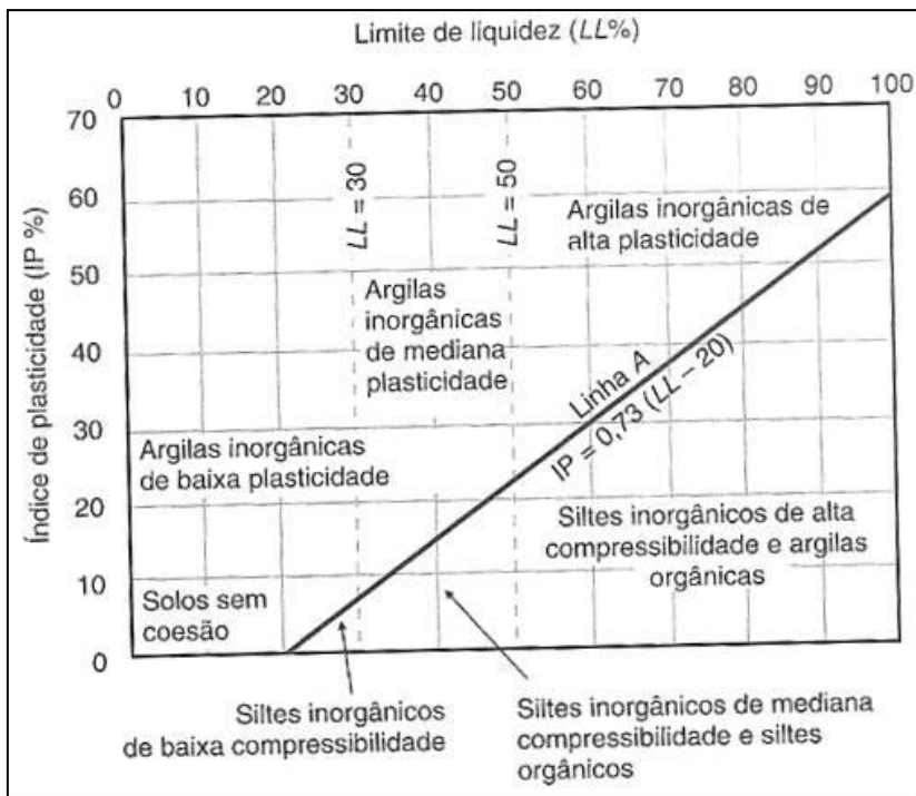
Figura 4 - Gráfico de plasticidade de Casagrande
