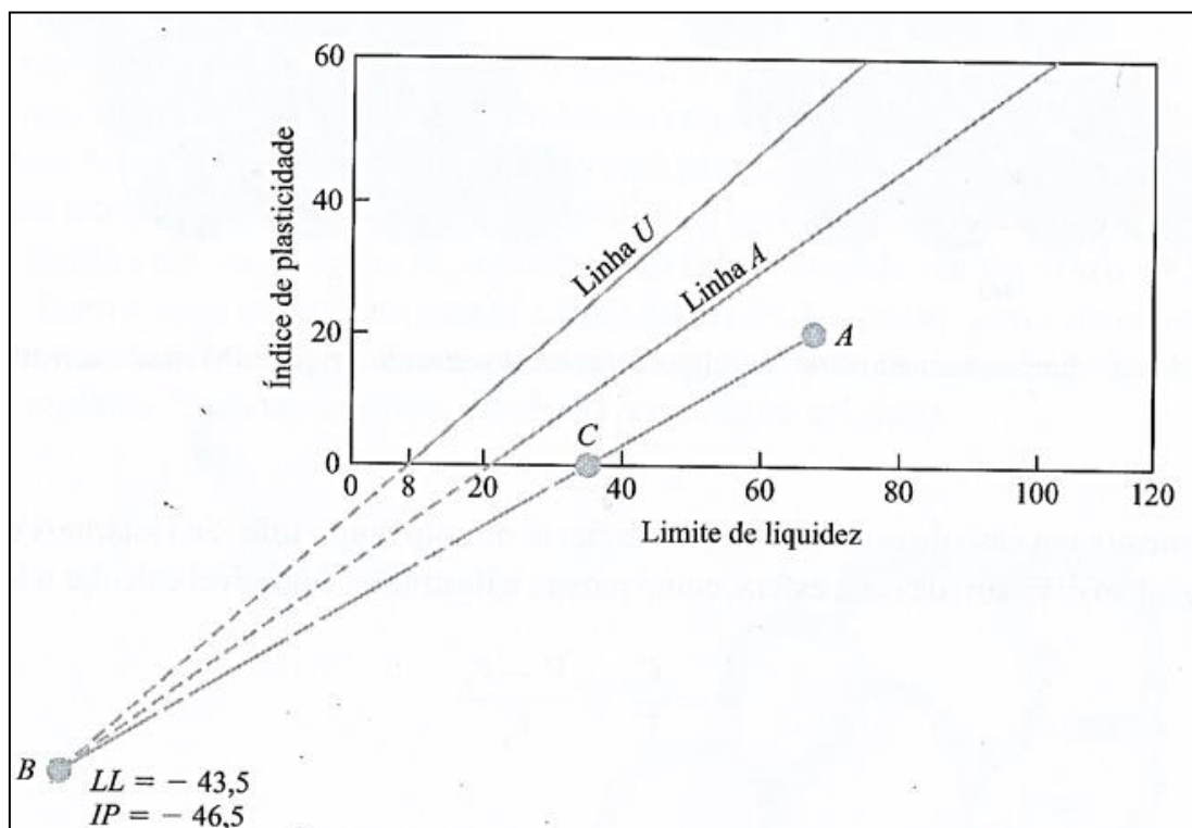
Figura 6 - Estimativa de contração com base no gráfico de plasticidade
